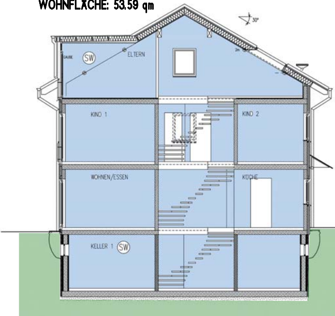
SCHNITT (Kellergeschoss als Sonderwunsch möglich)
