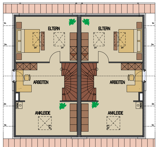
DACHGESCHOSS WOHNFLÄCHE: 31,85 qm
