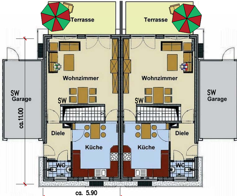
ERDGESCHOSS WOHNFLÄCHE: 53.34 qm
